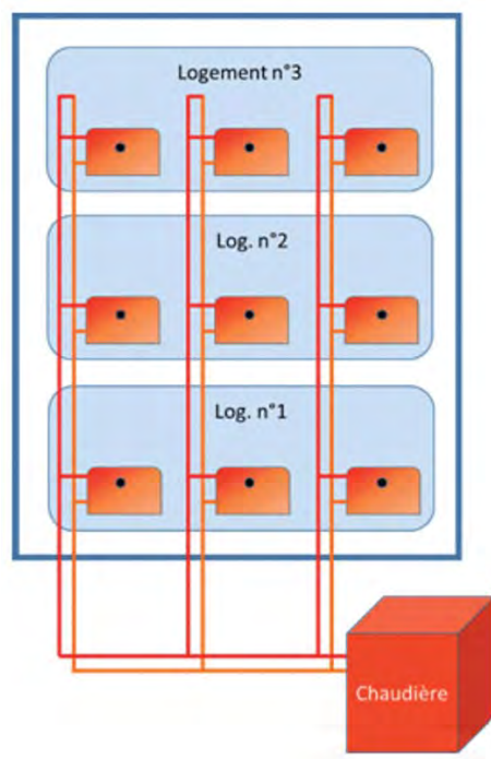
Schéma n°2 : réseau vertical avec emplacement des répartiteurs (points noirs) et exemple de répartiteur
